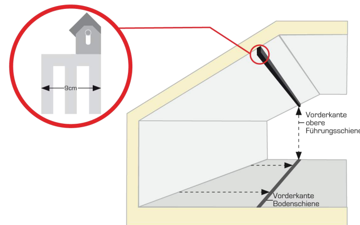
Seitenansicht
